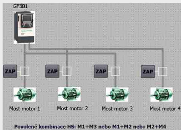
HAVARIJNÍ STRATEGIE - pojezdu mostu jeřábu Obrazovka z operačního panelu Siemens umístěného na rozvaděči jeřábu.
